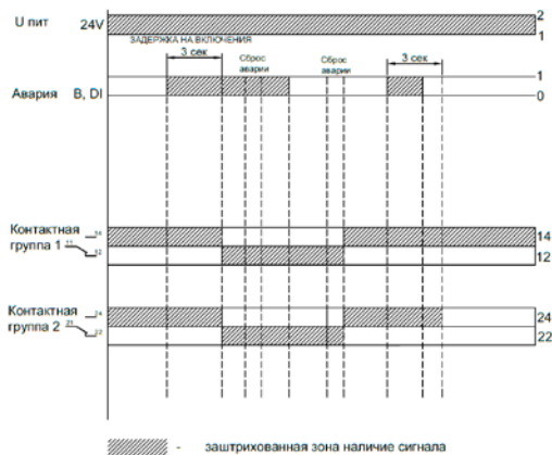
ДИАГРАММА РАБОТЫ RSA-B
