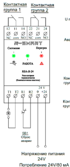
СХЕМА ПОДКЛЮЧЕНИЯ RSA-B
